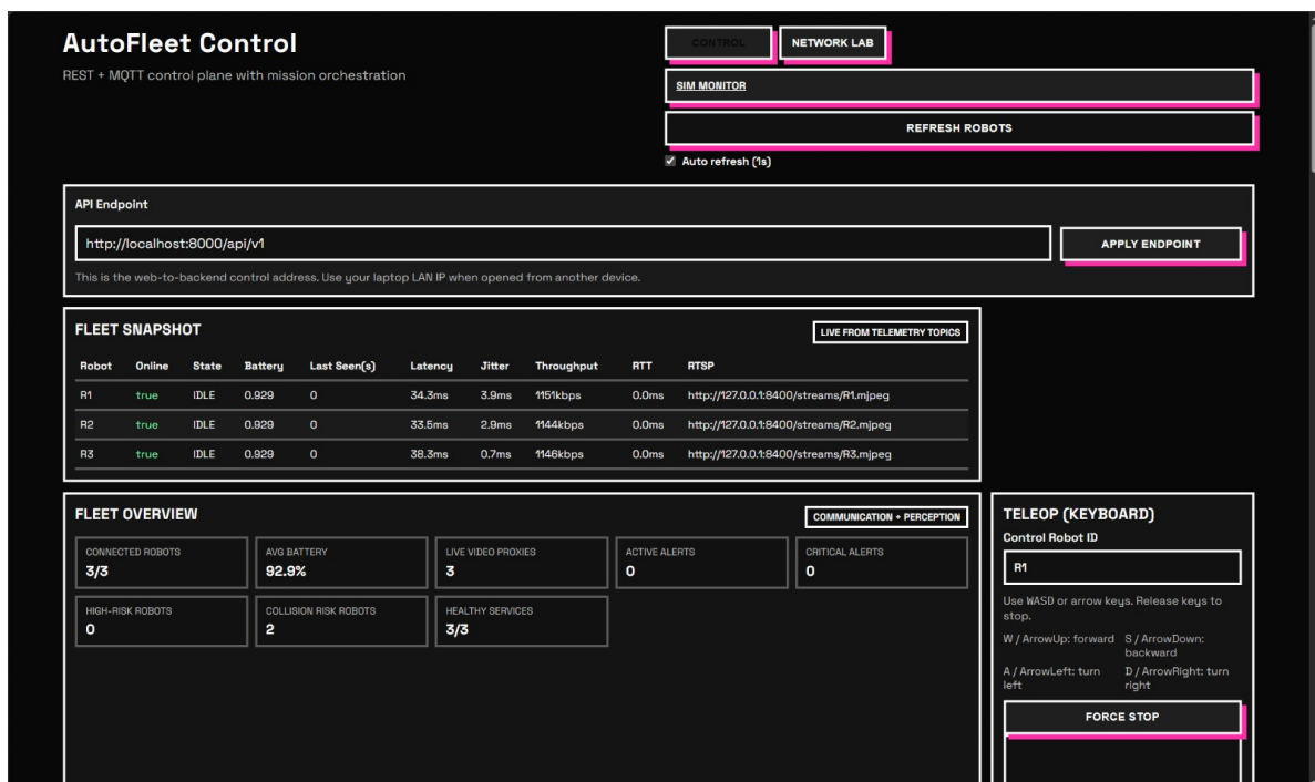
FIGURE 5.3 – Vue de diagnostic réseau et de gestion des flux vidéo
