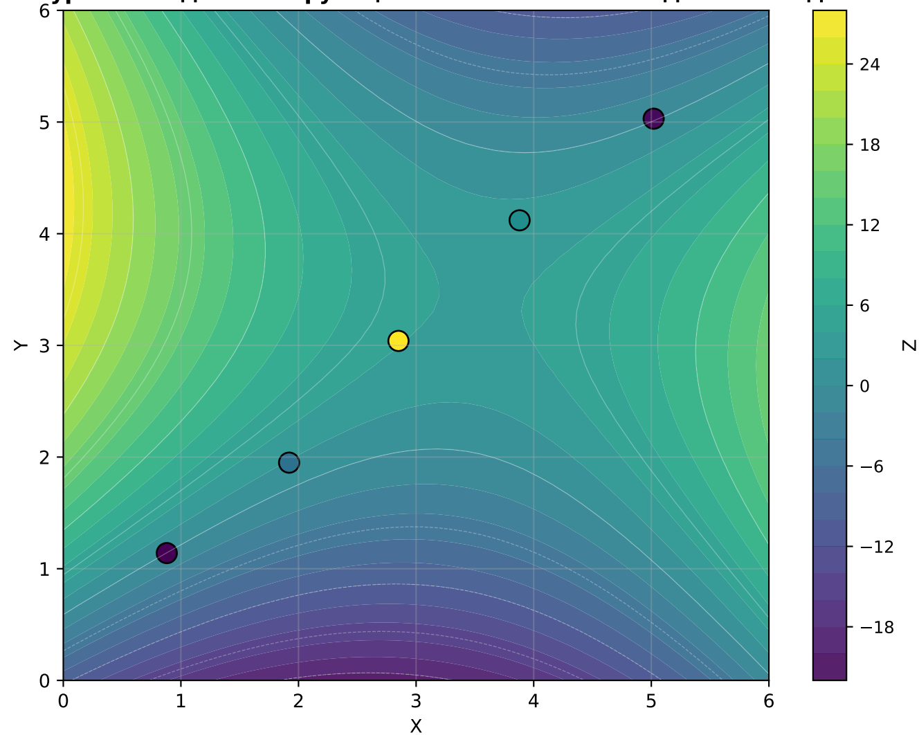
Линии уровня модельной функции и точки области задания исходной
