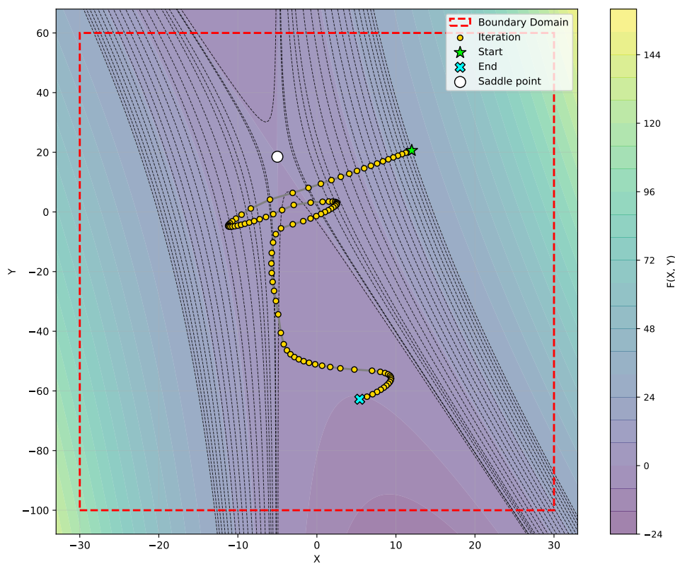
Рис. 3: Диаграмма последовательных пилообразных приближений Adam.
