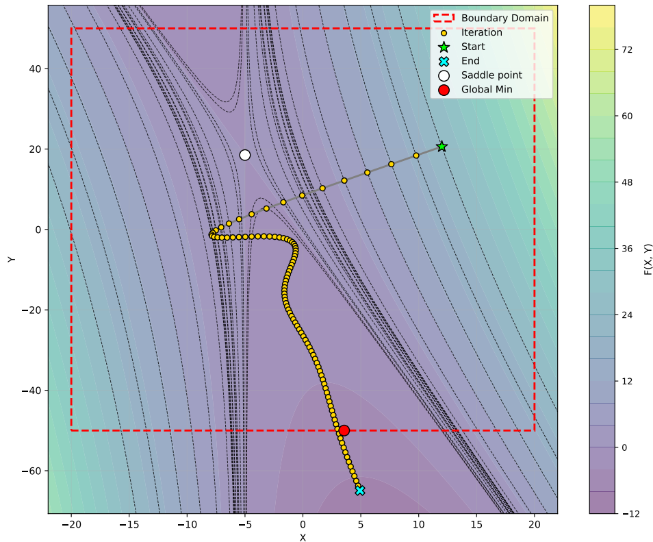
Рис. 3: Диаграмма последовательных приближений алгоритмом Adam.
