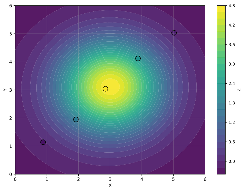
Рис. 14: Линии уровня RBF-сети после обучения.
