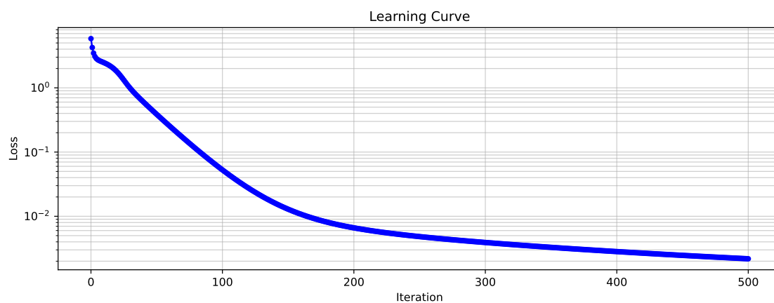
Рис. 11: Кривая обучения для RBF-сети.
