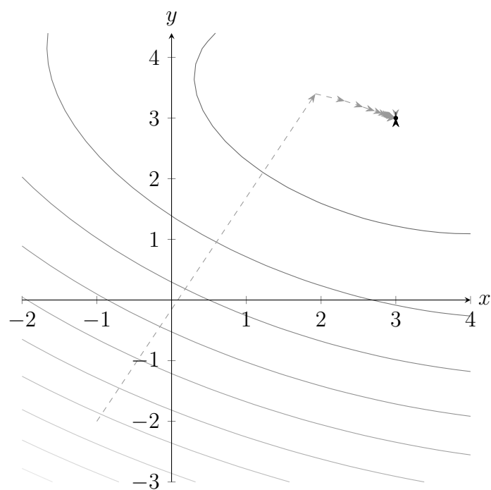
Рис. 8: Все итерации метода градиентного спуска.
