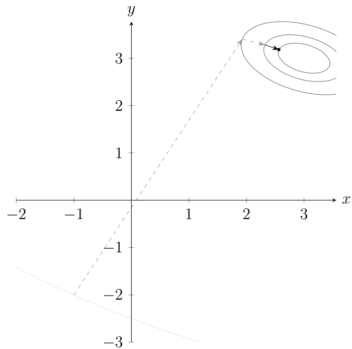
Рис. 7: Итерация №3 метода градиентного спуска.
