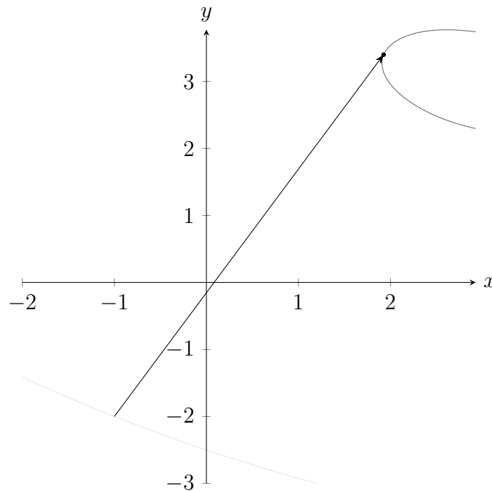
Рис. 5: Итерация №1 метода градиентного спуска.
