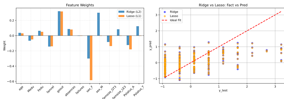
Рис. 4: Сравнение весов признаков и качества предсказаний.
