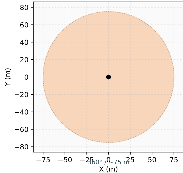
Waymo
