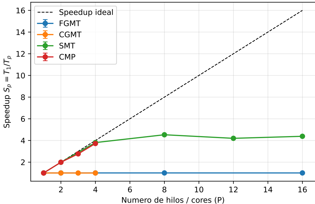
Caso 1: Speedup vs P (multiplicacion de matrices por bloques)
