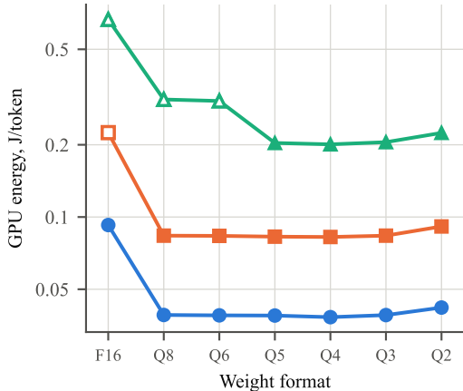
Prefill (prompt)
