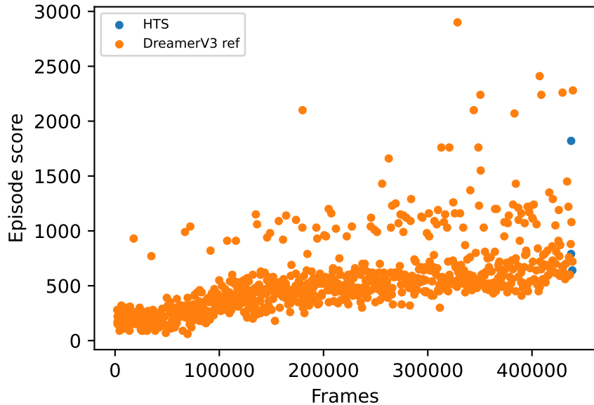
Alien
