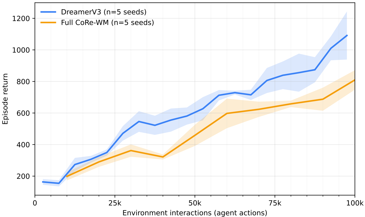
Qbert
