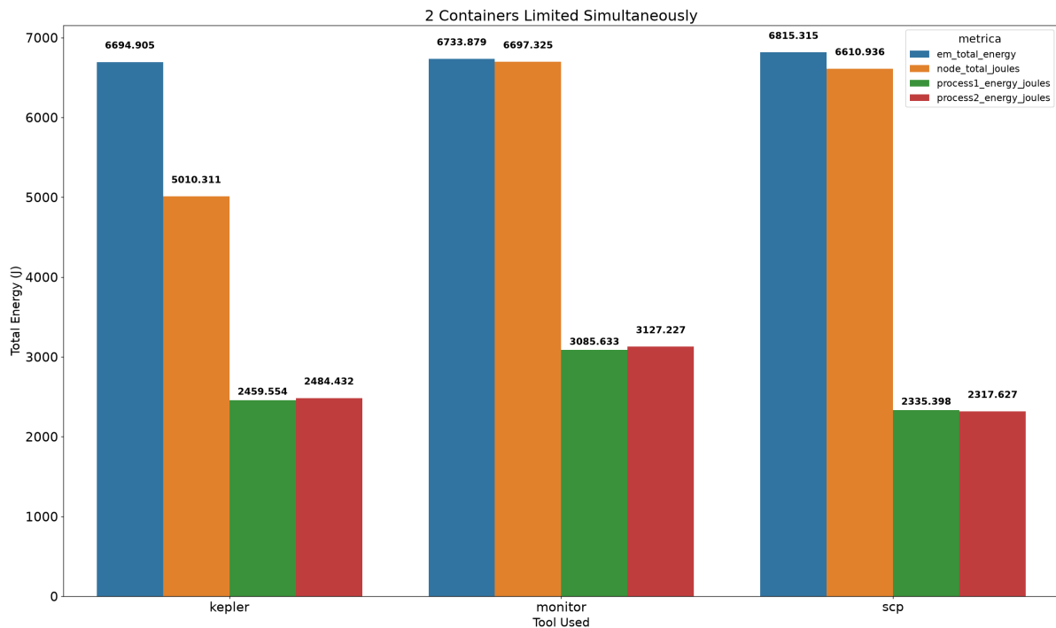
Figura 5.4: Histograma resultante de las metricas de consumo de dos contenedores limitados a 3 cores cada uno ejecutando tareas de codificacion simultaneamente
