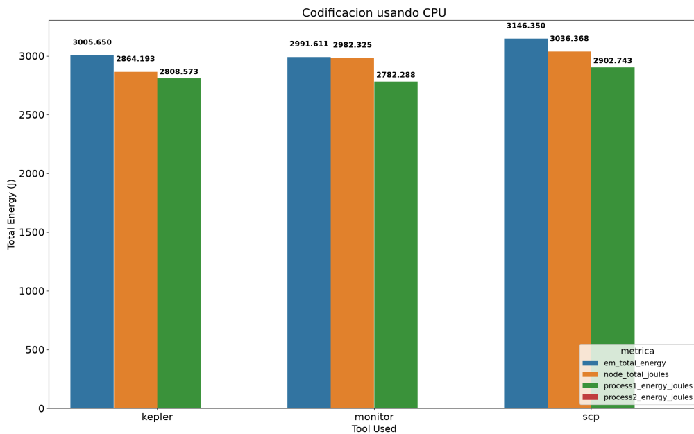
Figura 5.2: Histograma comparativo de las metricas de consumo energetico en julios de las tres herramientas en una tarea de codificacion empleando exclusivamente la CPU
