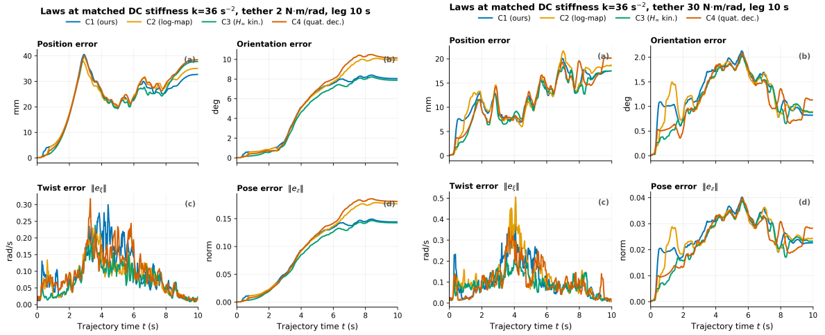
图 3: 等控制资源条件下的四律对比 ( k=36 , 单次运行, 10 s 标准轨迹): 左为 K_{tr}=2 \text{ N·m/rad} (拴定近乎退出的纯度极限, 准静态残差由摩擦死区决定、约 32–40 mm); 右为 K_{tr}=30 \text{ N·m/rad} (终态 \approx 17 \text{ mm} )。拴定刚度跨越一个数量级, 所示记录中的四条曲线接近; C1 的收益在证书 (表 1) 而非精度。
