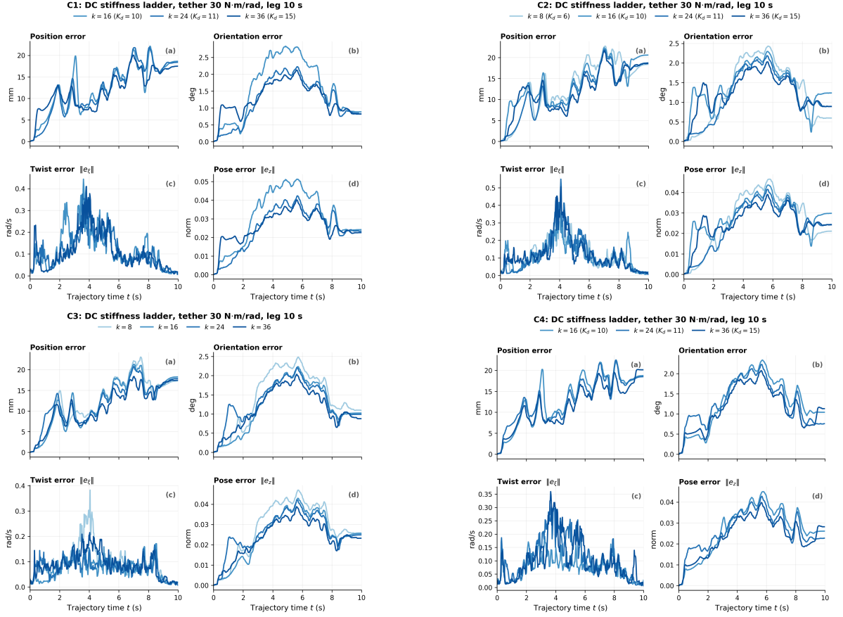
图 1: 各律增益阶梯 (拴定 30 \text{ N m/rad} , k \in \{8, 16, 24, 36\} 中各律可用档, 10 \text{ s} 标准轨迹单次运行, \text{traj\_t} 对齐): 姿态与 twist 瞬态误差随 k 单调下降, 位置误差弱下降, 与 \gamma^* 收紧 (定理 3(c')) 的方向一致。
