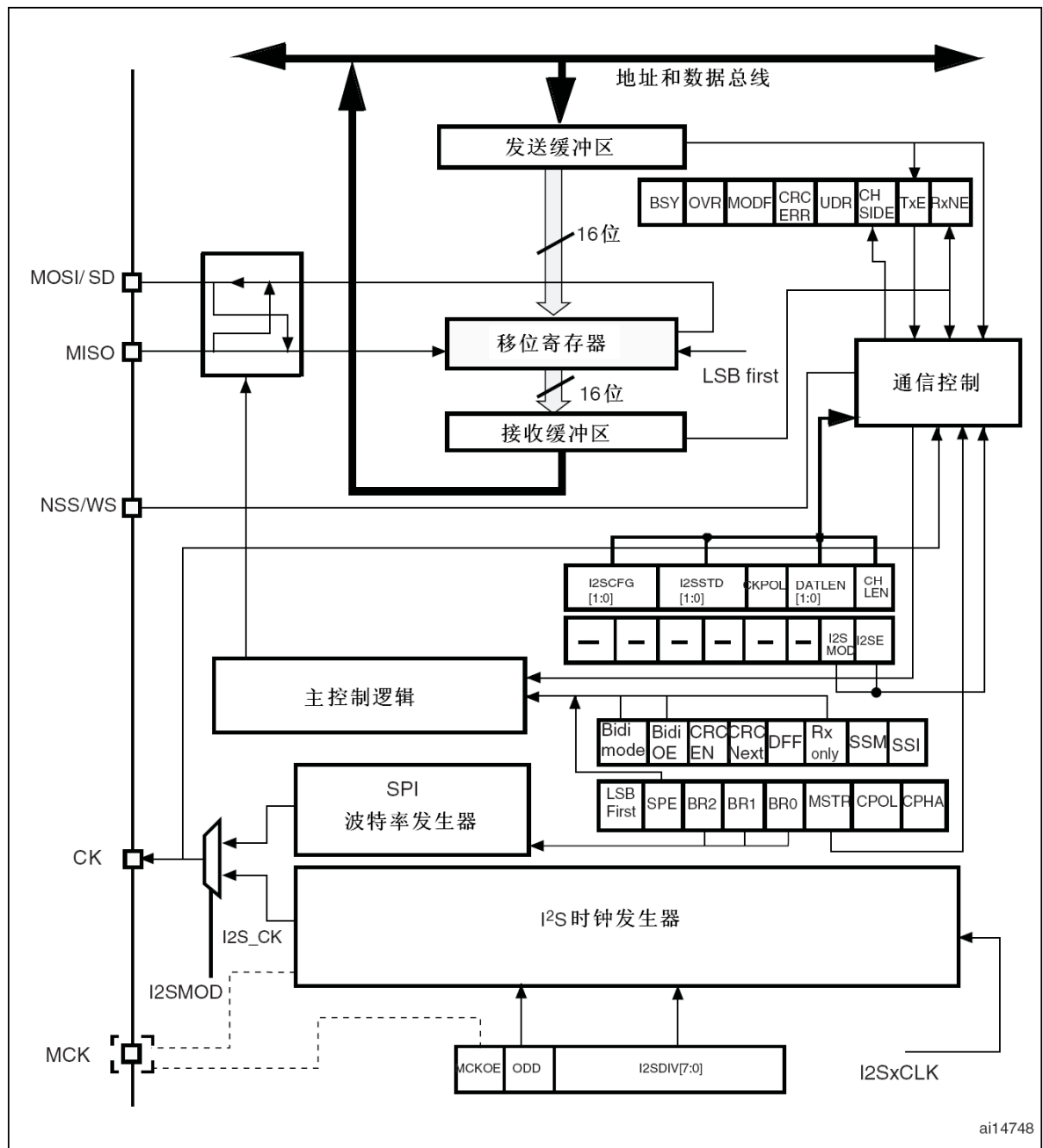
图221 I^2S 框图
