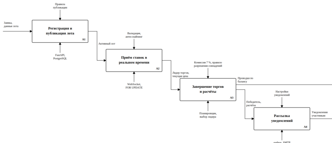
Рисунок 1.3 – Декомпозиция целевого процесса (IDEF0, A0)
