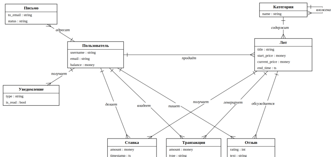
Рисунок 1.7 – Концептуальная модель данных (ER-диаграмма)
