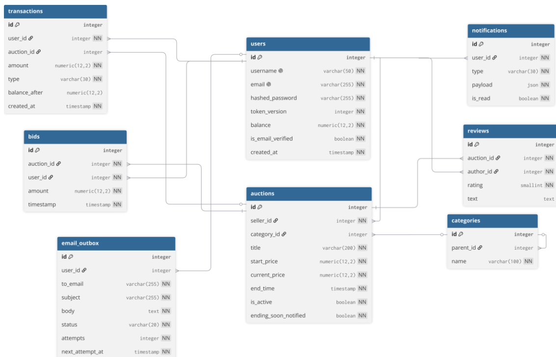
Рисунок 2.2 – ER-диаграмма базы данных
