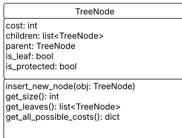
Abbildung 7: TreeNode Klasse
