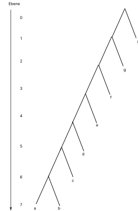
Abbildung 5: Ausgearteter Baum
