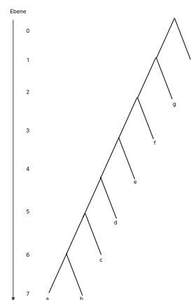
Abbildung 5: Ausgearteter Baum
