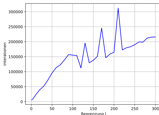
Abbildung 24: Iterationen labyrinth8.txt
