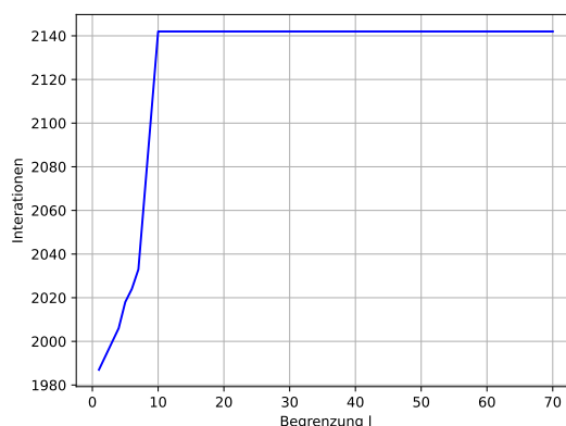
Abbildung 22: Iterationen labyrinth6.txt
