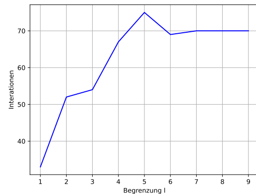
Abbildung 12: Iterationen labyrinth1.txt
