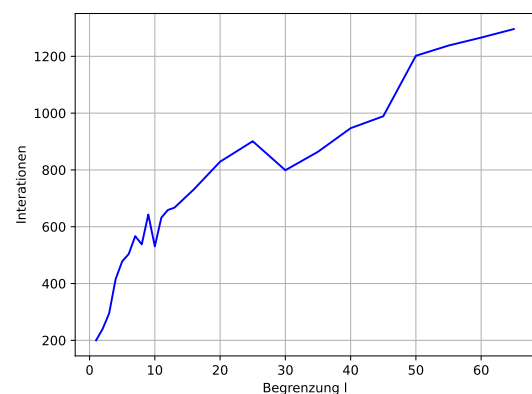
Abbildung 16: Iterationen labyrinth3.txt
