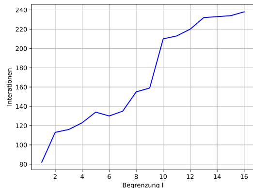
Abbildung 14: Iterationen labyrinth2.txt
