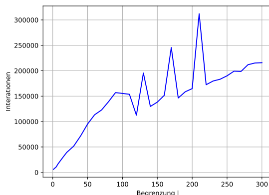
Abbildung 24: Iterationen labyrinth8.txt
