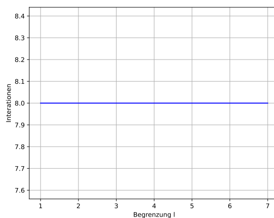
Abbildung 10: Iterationen labyrinth0.txt
