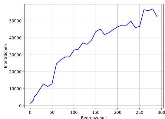
Abbildung 26: Iterationen labyrinth9.txt
