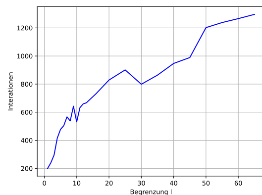
Abbildung 16: Iterationen labyrinth3.txt
