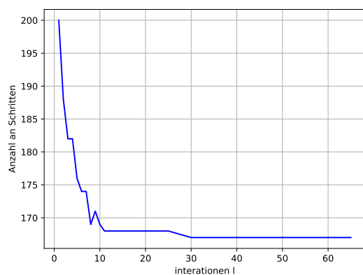
Abbildung 15: Genauigkeit labyrinth3.txt
