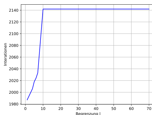
Abbildung 22: Iterationen labyrinth6.txt
