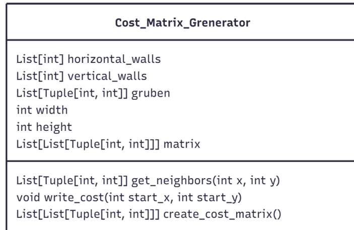
Abbildung 11: Klasse Cost_Matrix_Generator
