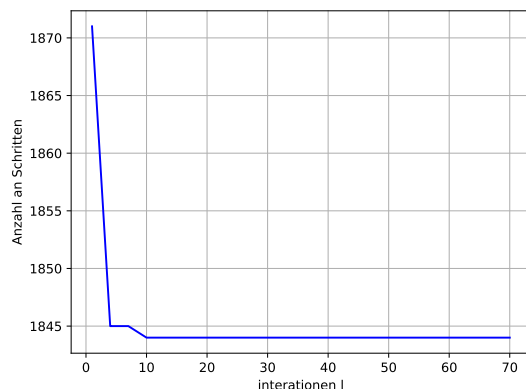
Abbildung 21: Genauigkeit labyrinth6.txt
