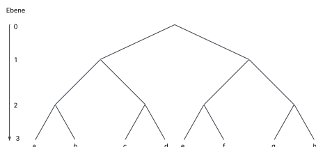
Abbildung 2: Balancierter Baum
