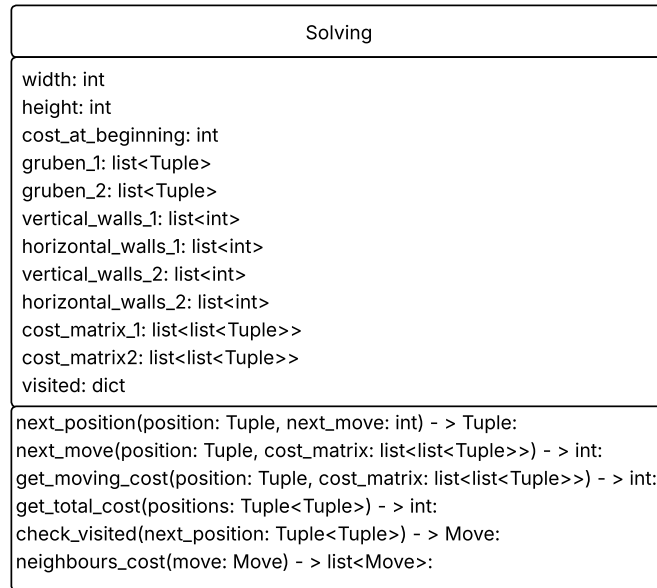
Abbildung 12: Solving Klasse
