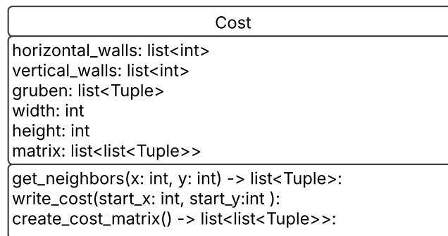
Abbildung 11: Cost Klasse
