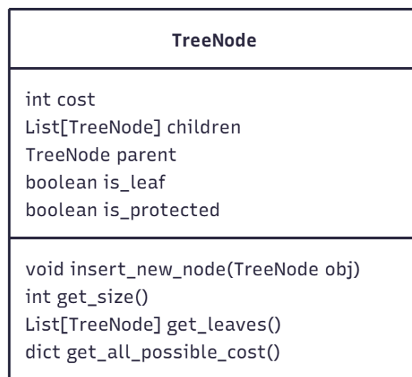
Abbildung 7: Klasse TreeNode
