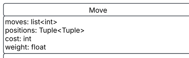
Abbildung 13: Move Klasse
