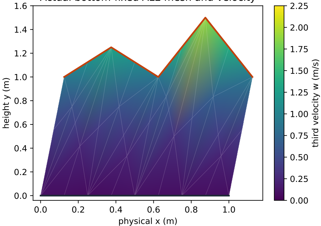
Actual bottom-fixed ALE mesh and velocity
