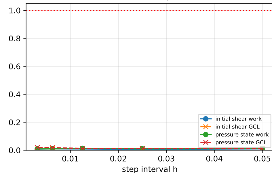
Actual defect / unchanged allowance
