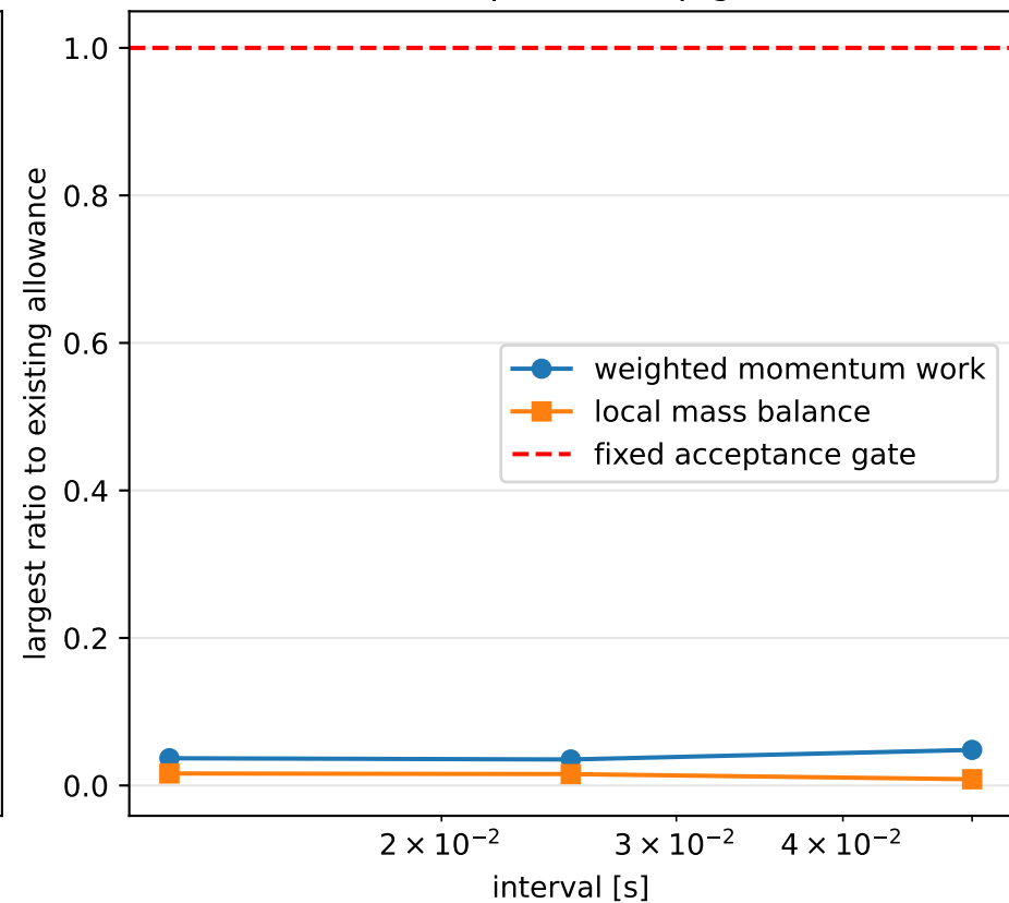
Actual repeated-step gates
