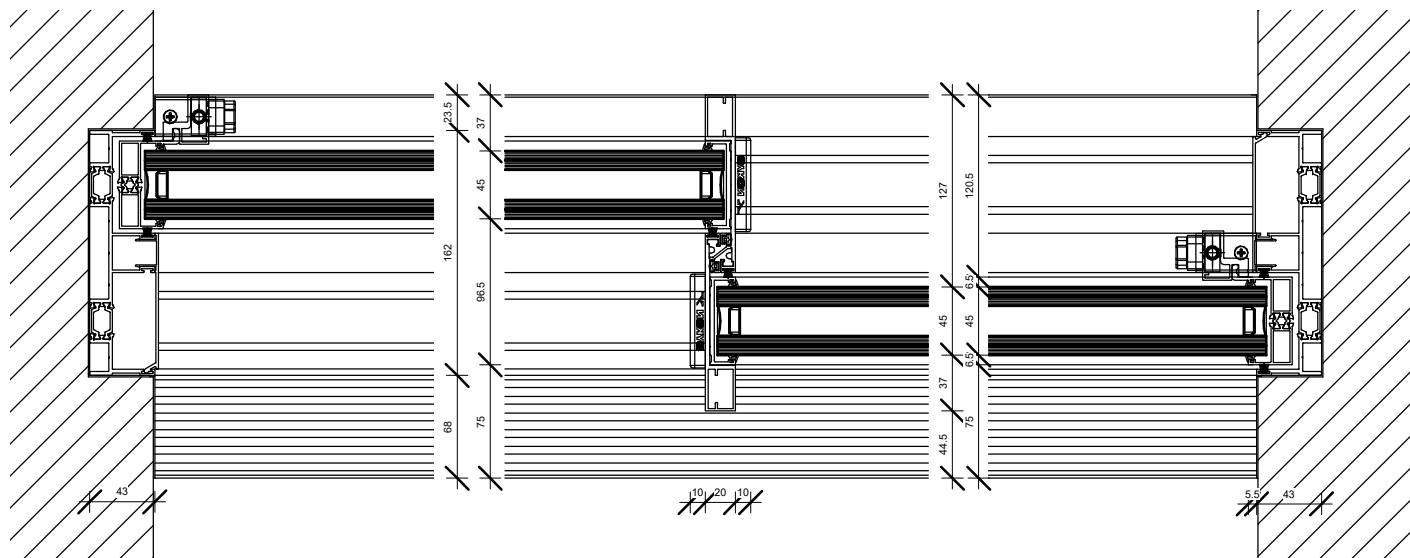
3 Detail 1 1 : 5
