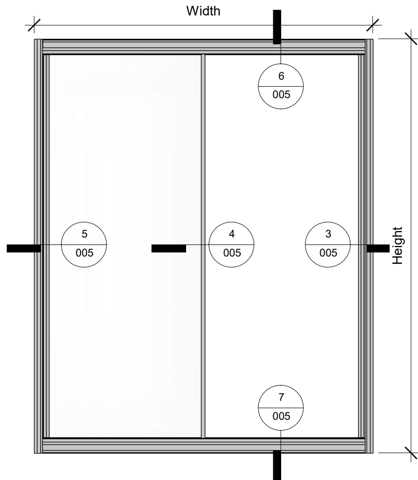
2 Elevation Back 1 : 20
