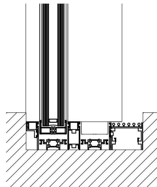
7 Detail 5 1 : 5
