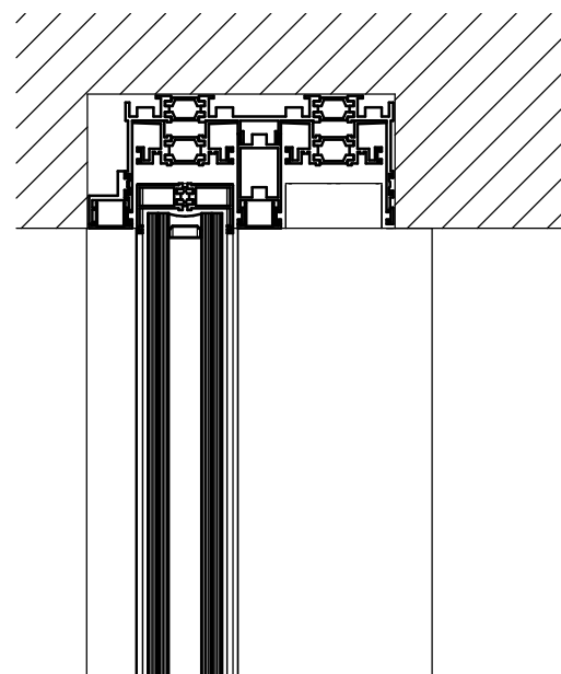
6 Detail 4 1 : 5
