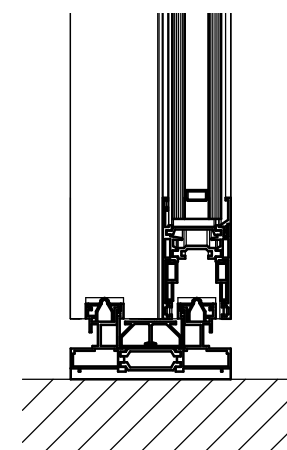
7 Detail 5 1 : 5
