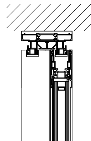
6 Detail 4 1 : 5
