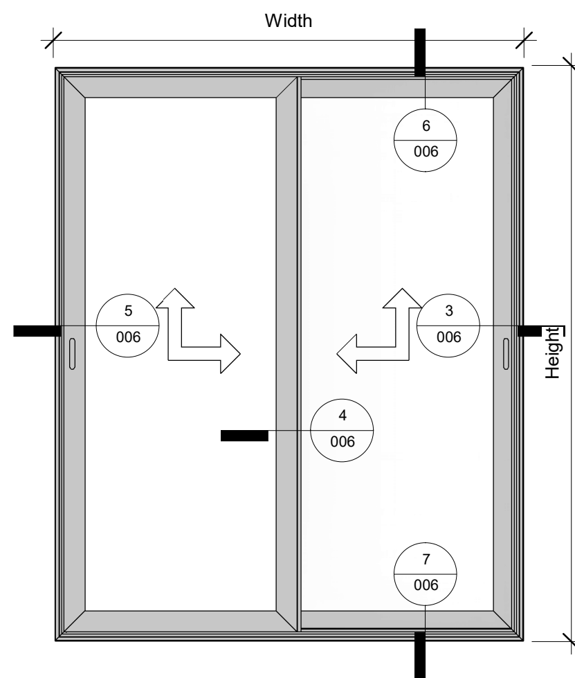
2 Elevation Back 1 : 20
