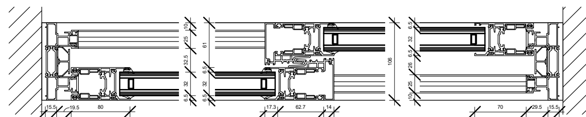
3 Detail 1 1 : 5
