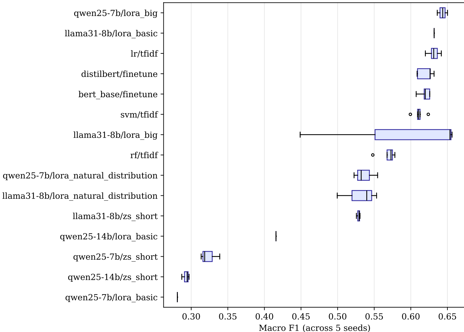
Wariancja po seedach — liar
