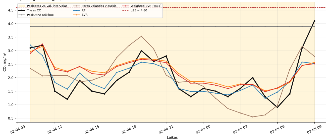
Tipinis geras: B_S1, kaukė 42, blokas 14
