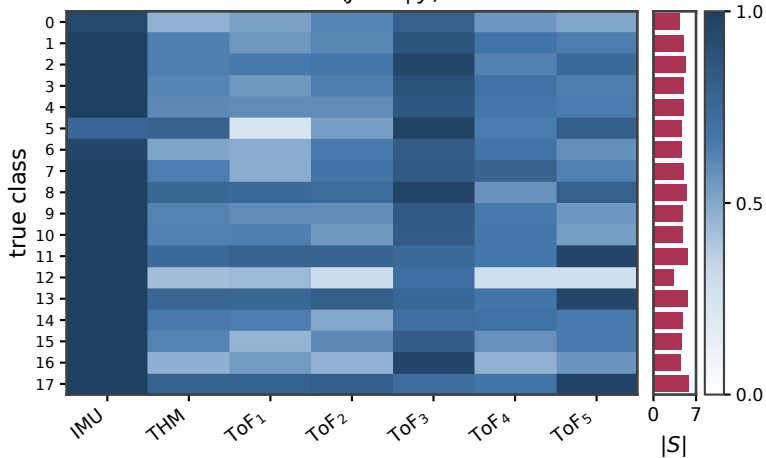
CMI P(j \in S | y)
