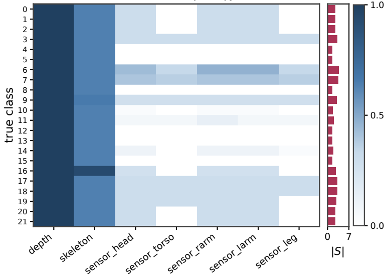
CZU-MHAD P(j \in S | y)
