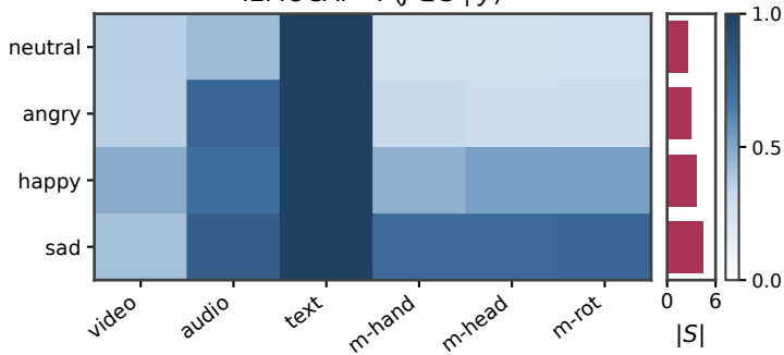
IEMOCAP P(j \in S | y)
