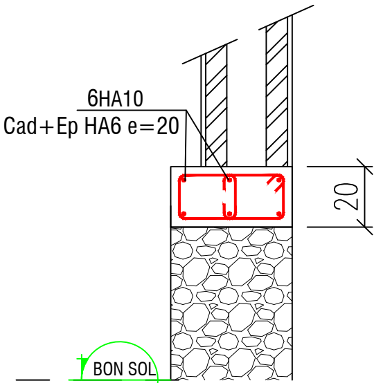
CH (40x20)
