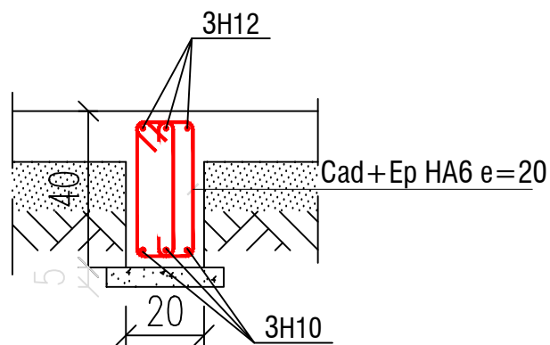
LG (20x40)
