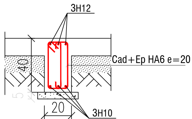
LG1 (20x50)
