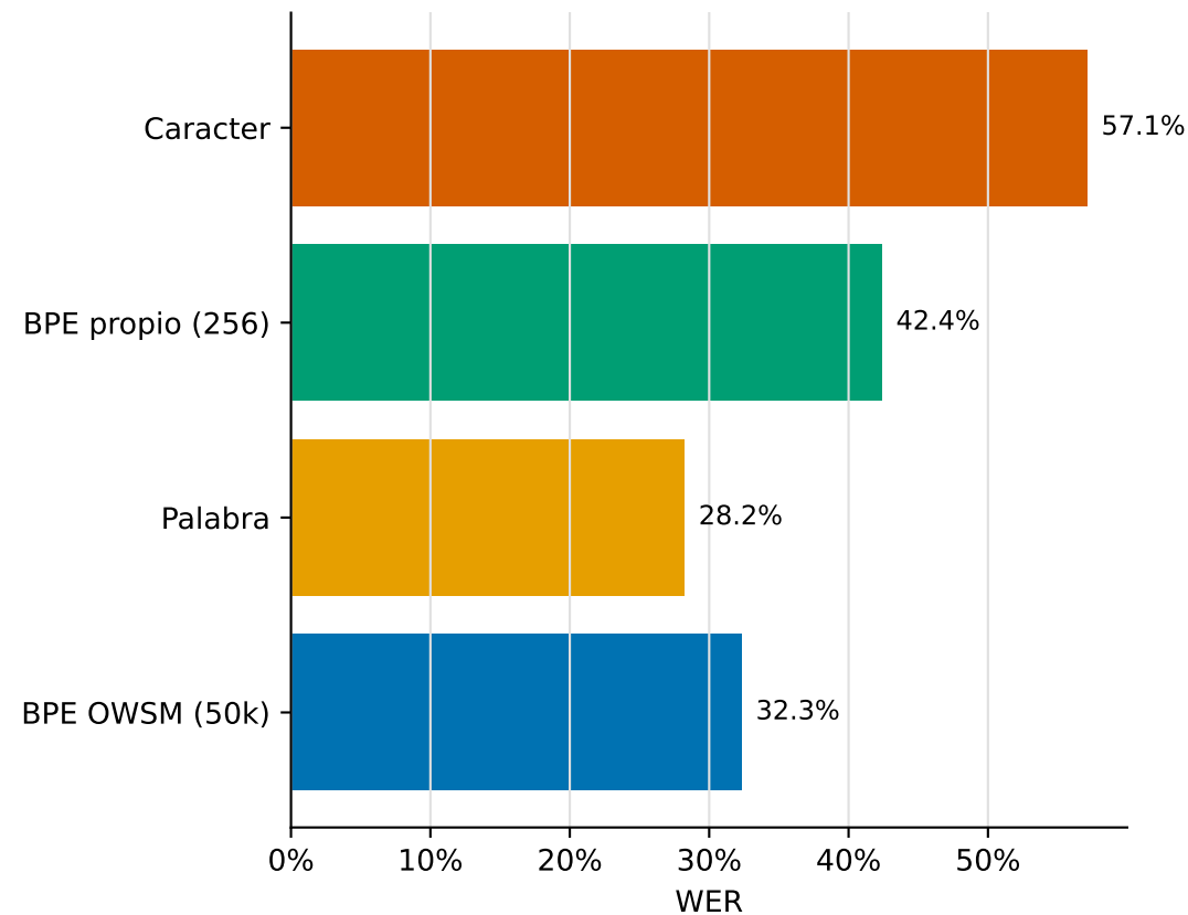
Rendimiento del texto reconstruido
