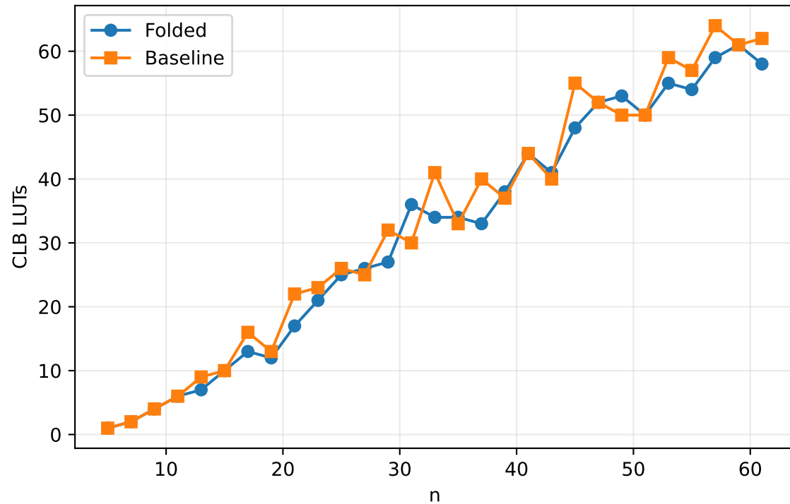
Vivado CLB LUT Count
