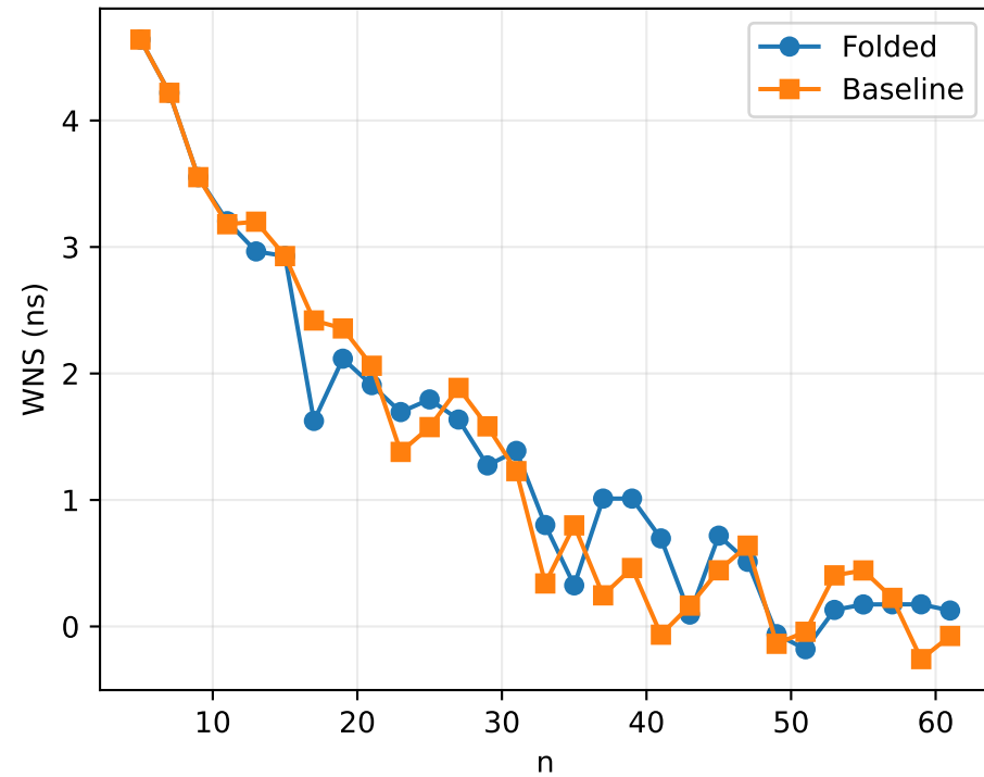
Worst Negative Slack
