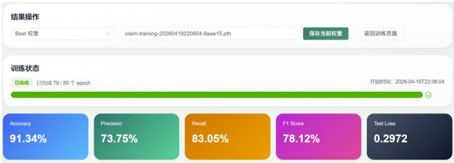
(a) 训练结果保存和摘要界面
