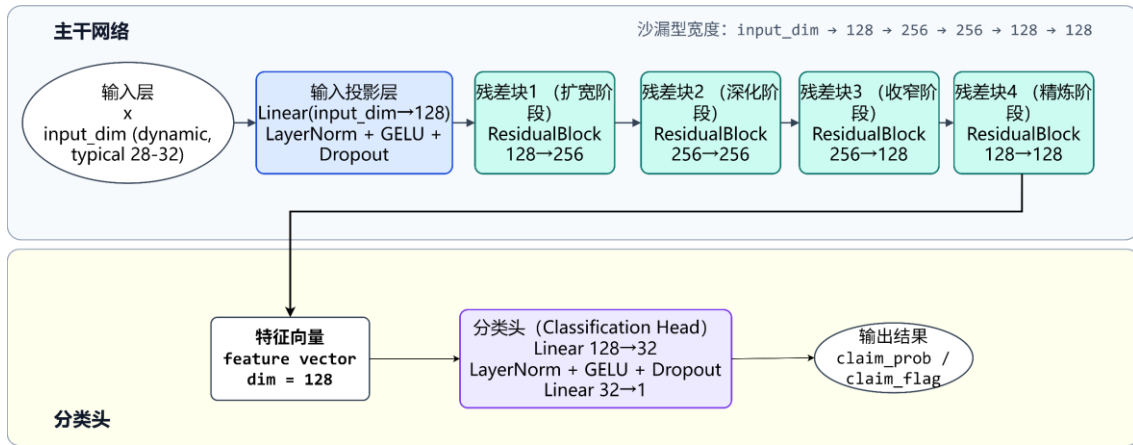
图 4.2 InsuranceMLP 网络结构图
