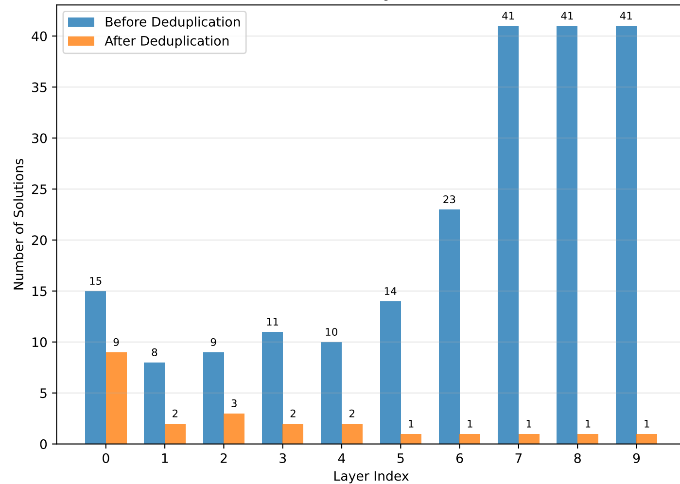
VGG16 - Array 512x512
