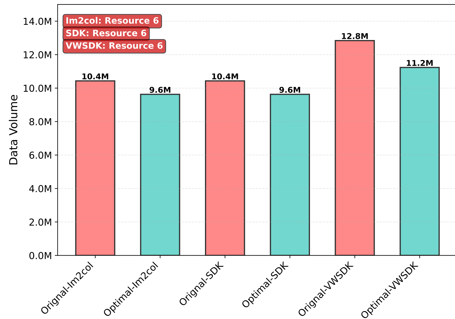
VGG16 (512*512)
