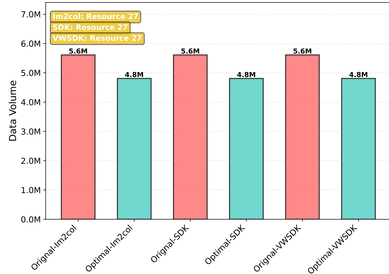
VGG16 (512*512)
