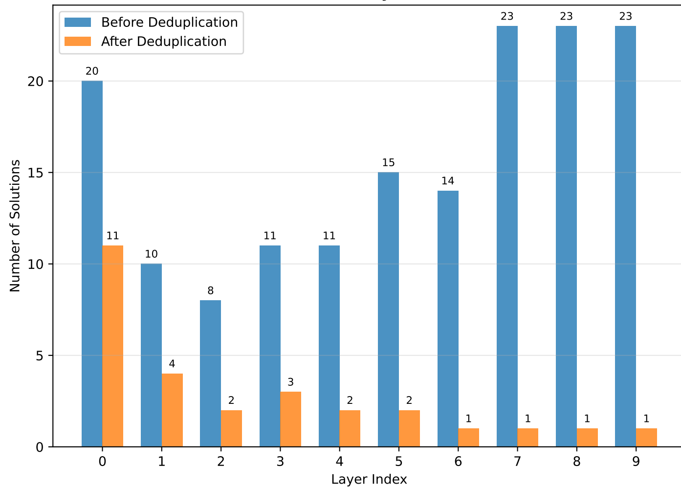
VGG16 - Array 256x512
