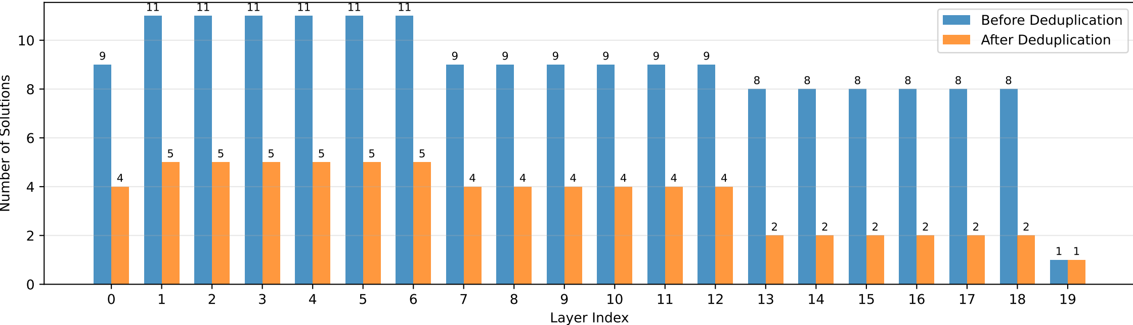
RESNET20 - Array 256x512
