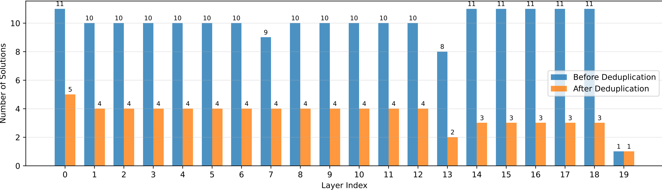
RESNET20 - Array 256x256
