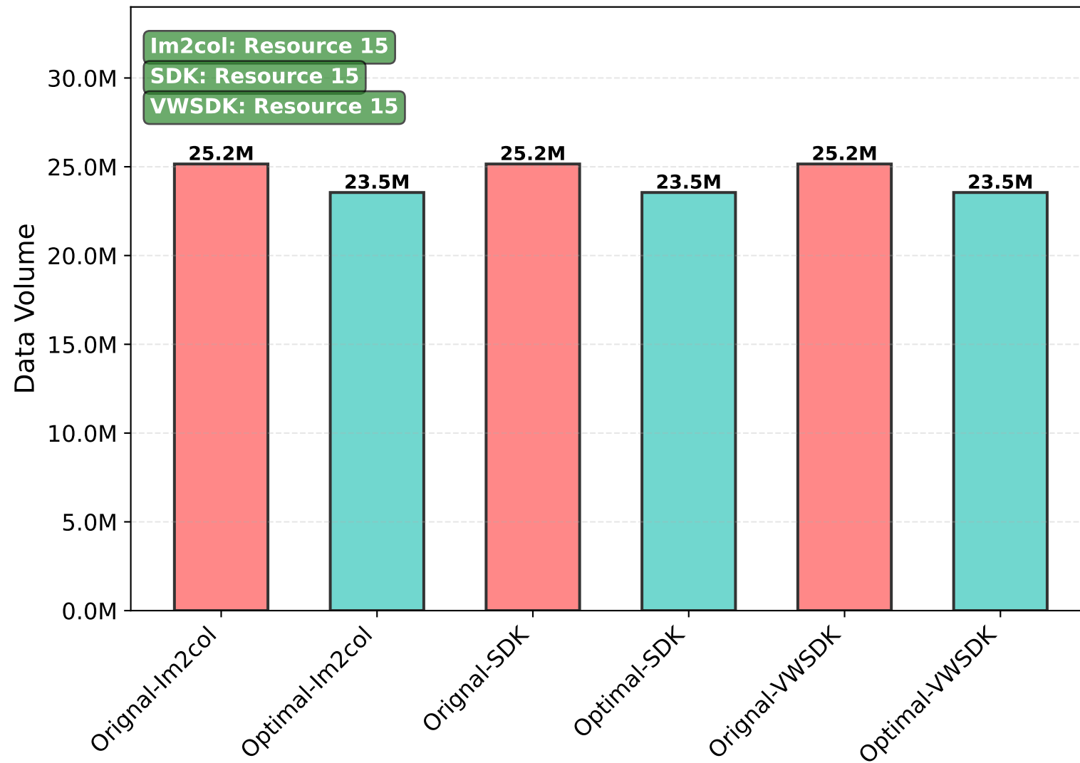
VGG16 (256*512)
