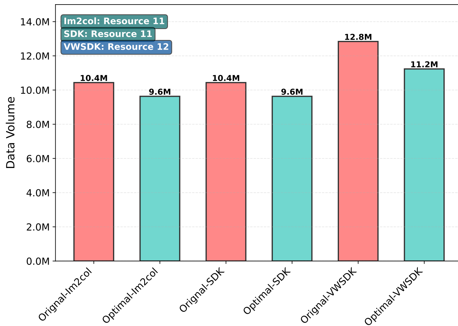
VGG16 (256*512)
