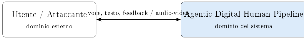
Figura 2: DFD livello 0.
