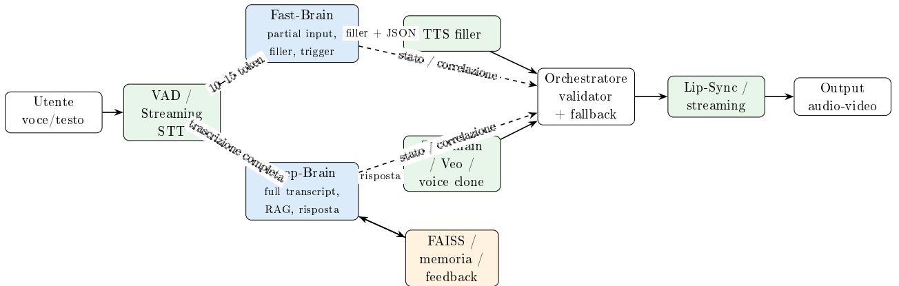
Figura 2: Pipeline agentic dual-brain analizzata.
