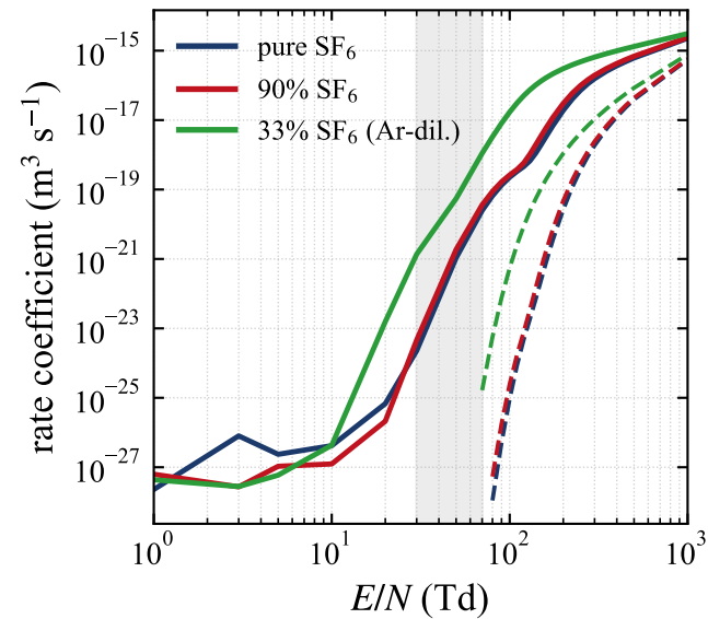
Ionization
