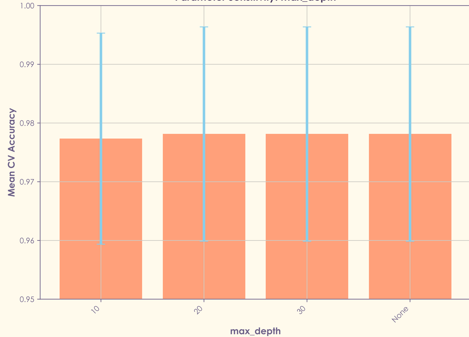
Parameter Sensitivity: max_depth
