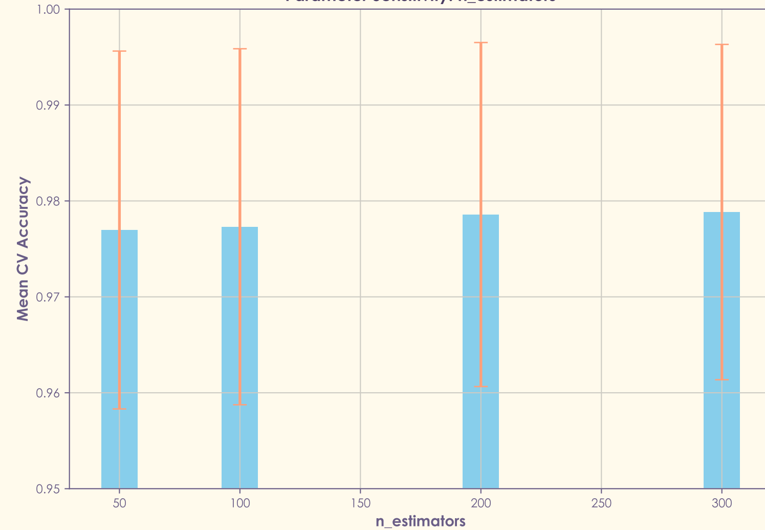
Parameter Sensitivity: n_estimators
