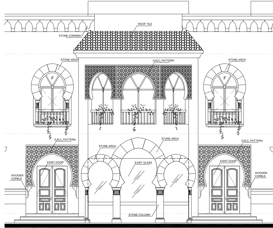
5 ENLARGED ELEVATION SCALE: 1:50 M. A120301
