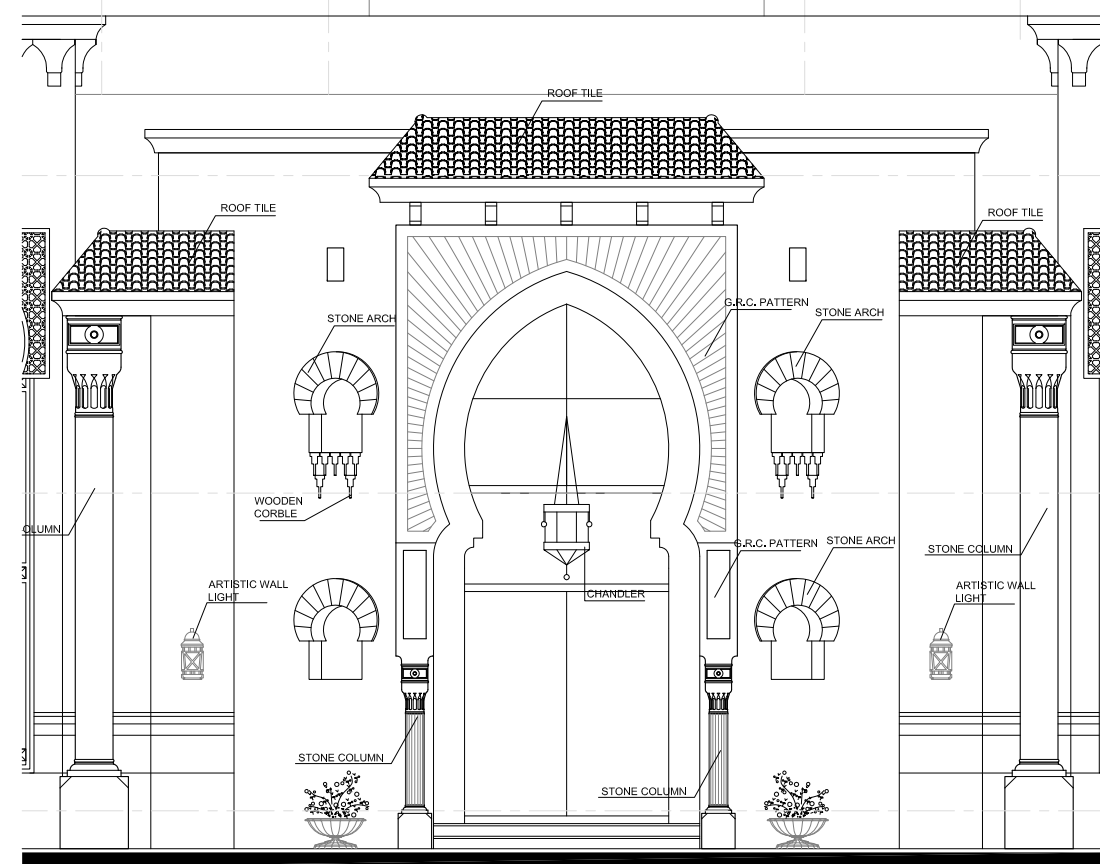
5 ENLARGED ELEVATION A120302 SCALE: 1:50 M.
