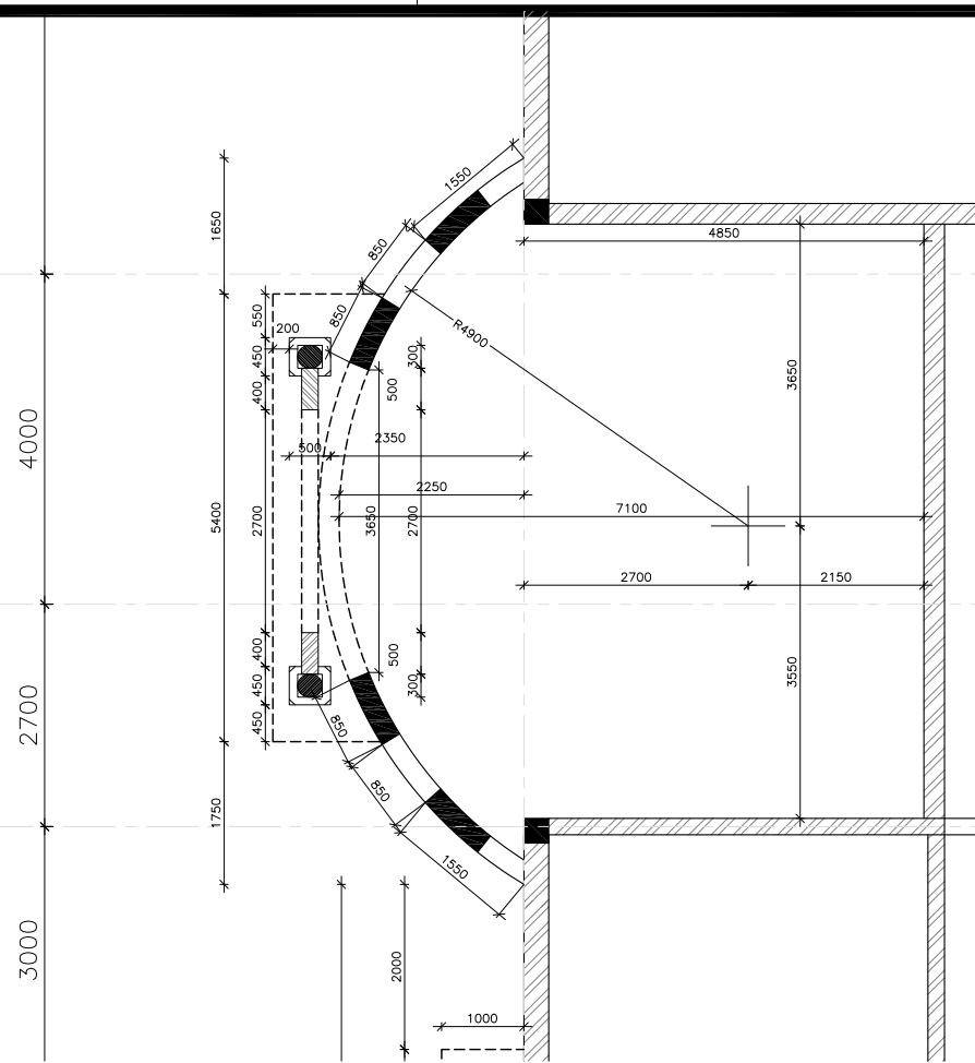
1 ENLARGED PLAN A120302 SCALE: 1:50 M.
