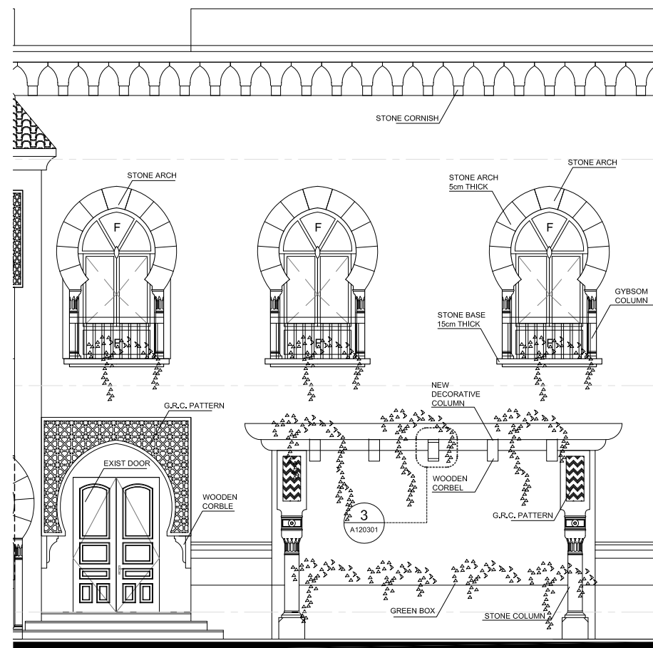
2 ENLARGED ELEVATION SCALE: 1:50 M. A120301
