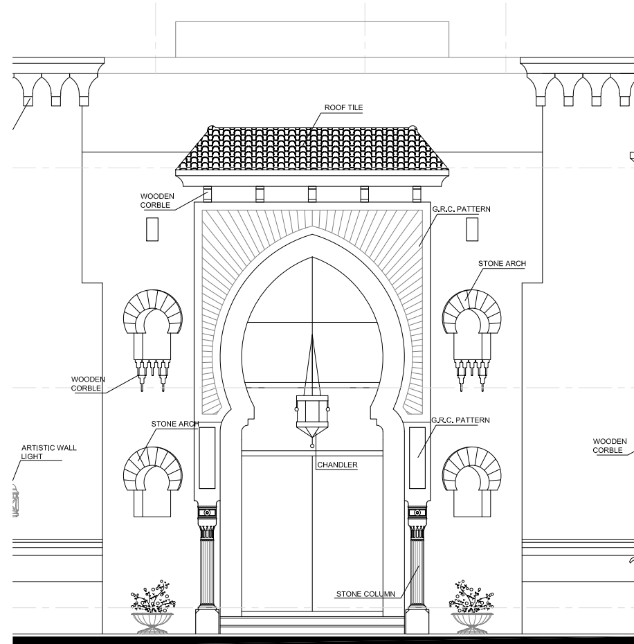
2 ENLARGED ELEVATION A120302 SCALE: 1:50 M.
