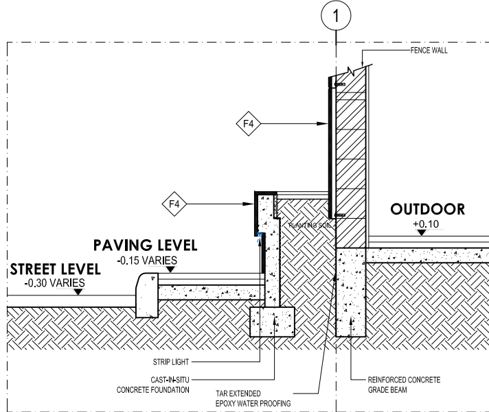
16 ARCH'L DETAIL
