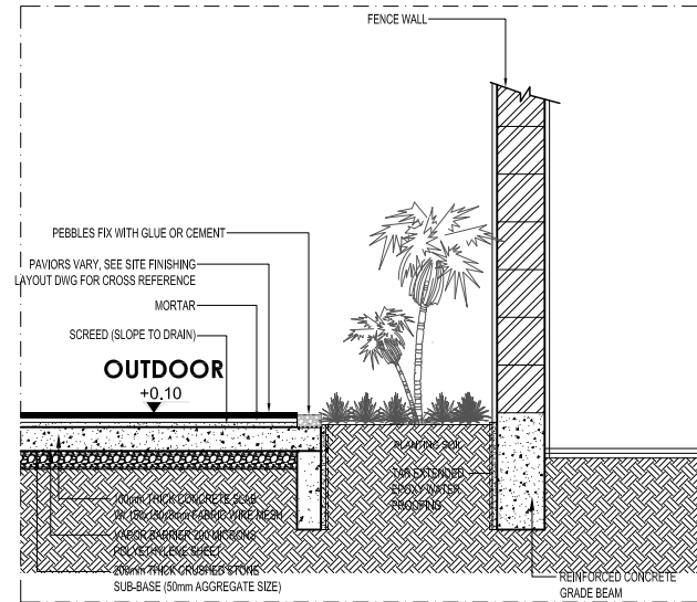
17 ARCH'L DETAIL
