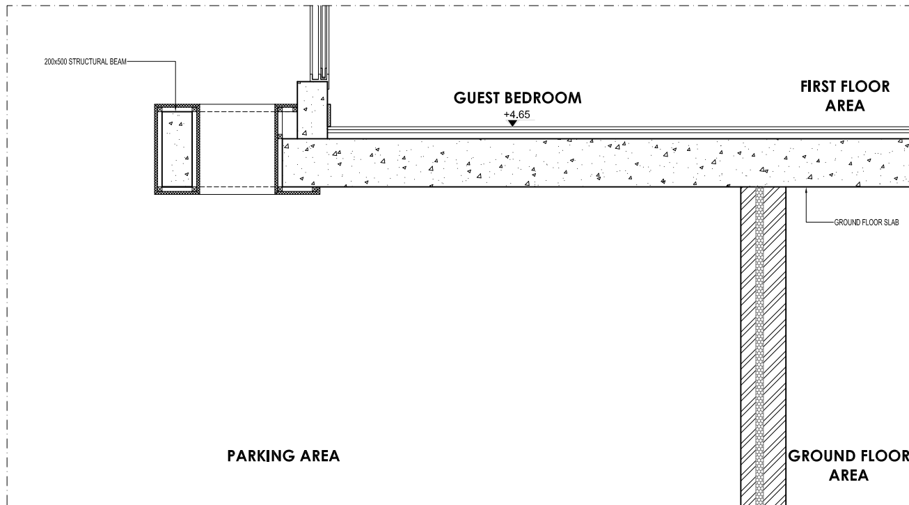
18 ARCH'L DETAIL
